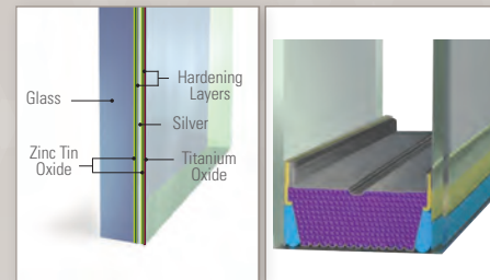
6 Layer Glass
